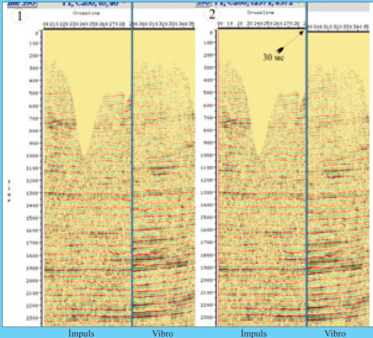
Şəkil 3. İmpuls və vibrasiya mənbələri üçün line 390 üzrə xam cəm kəsilişlər:
