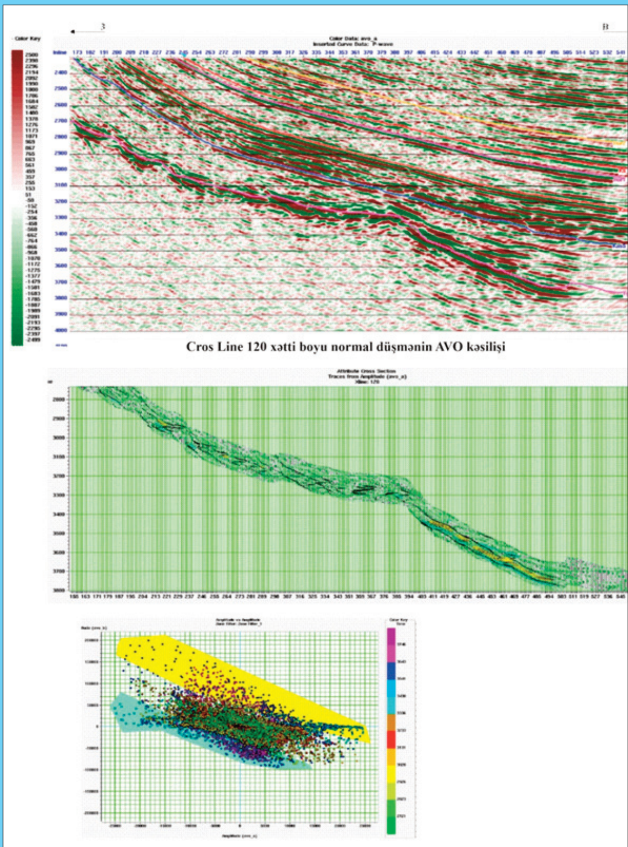
Şəkil 11. Cross Line 120 xətti boyu AVO-analizin nəticələri
