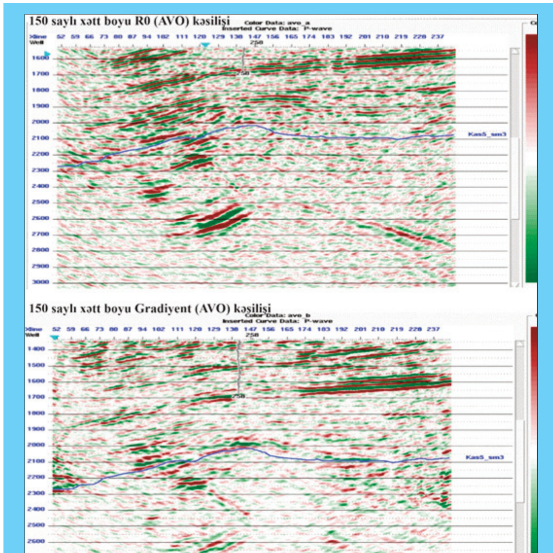
Şəkil 9. AVO-nun normal düşmə və qradient kəsilişləri
