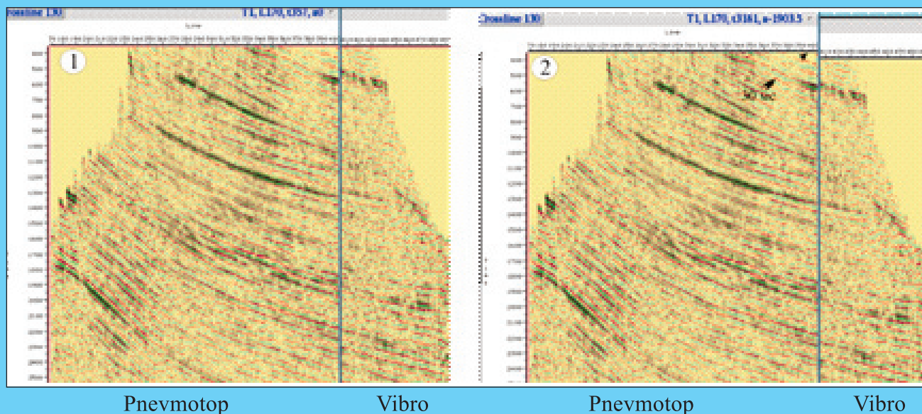
Şəkil 4. İmpuls və vibrasiya mənbələri üçün crossline130 üzrə xam cəm kəsilişlər:
