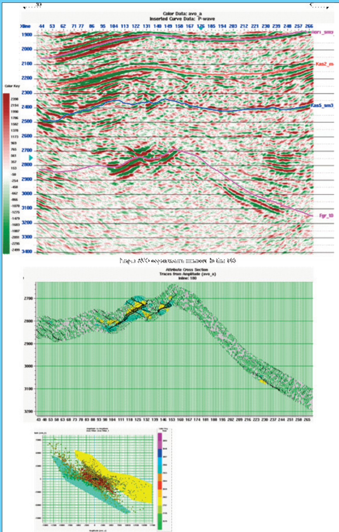
Şəkil 13. İn Line 180 xətti boyu AVO-analizin nəticələri
