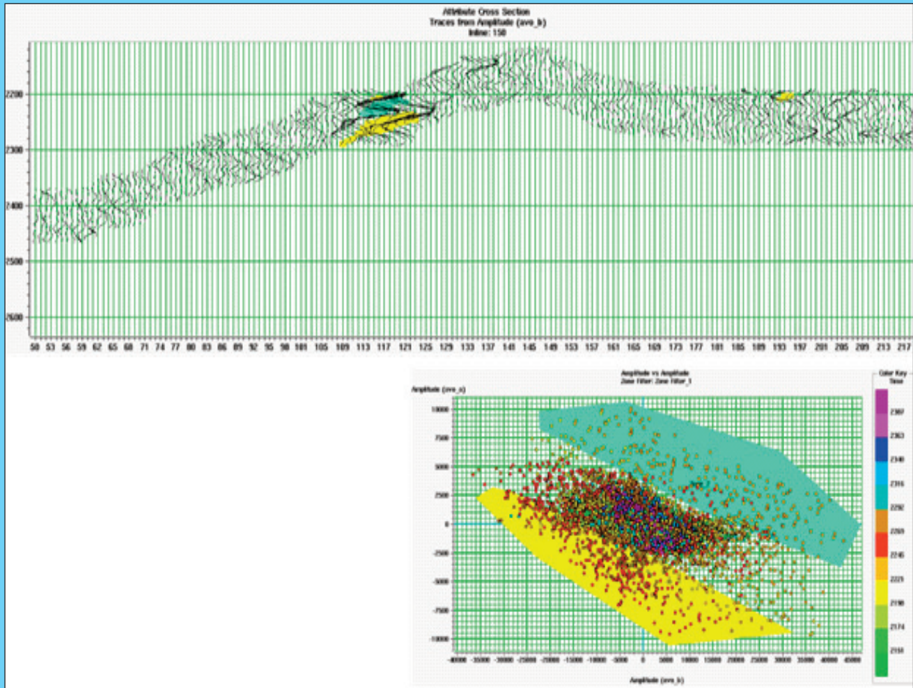
Şəkil 10. AVO - atributlarında anomaliyaların ayrılması
