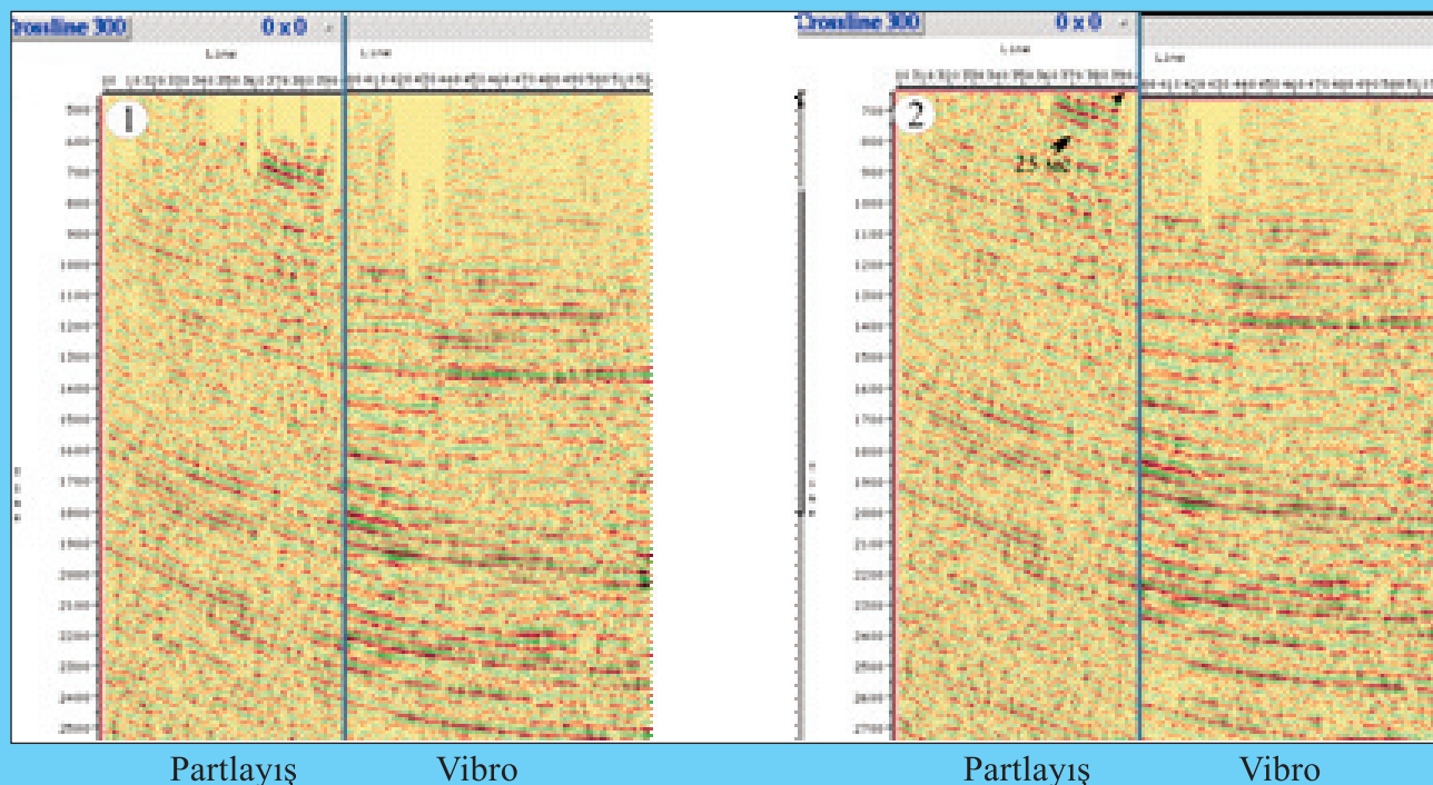
Şəkil 5. Partlayış və vibrasiya mənbələri üçün crossline 300 üzrə xam cəm kəsilişlər:
