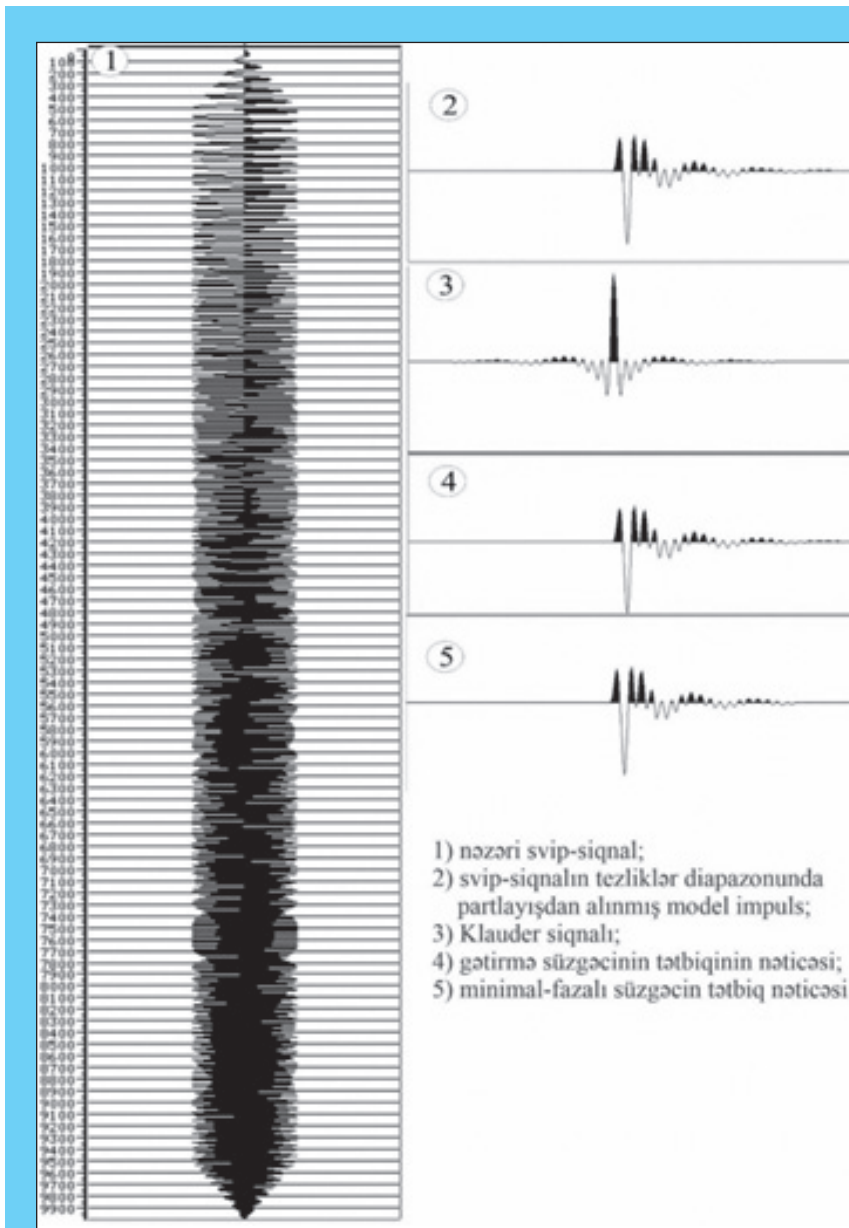
Şəkil 2. Modelləşdirmə vasitəsilə vibrasiya mənbəyinin signalının minimal-fazlı impuls formasına gətirilməsi
