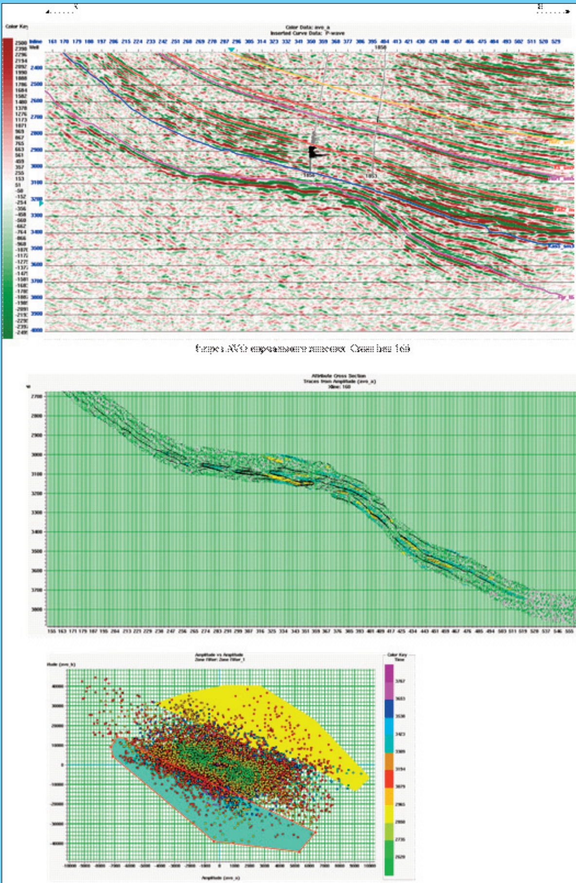
Şəkil 12. Cross Line 160 xətti boyu AVO-analizin nəticələri
