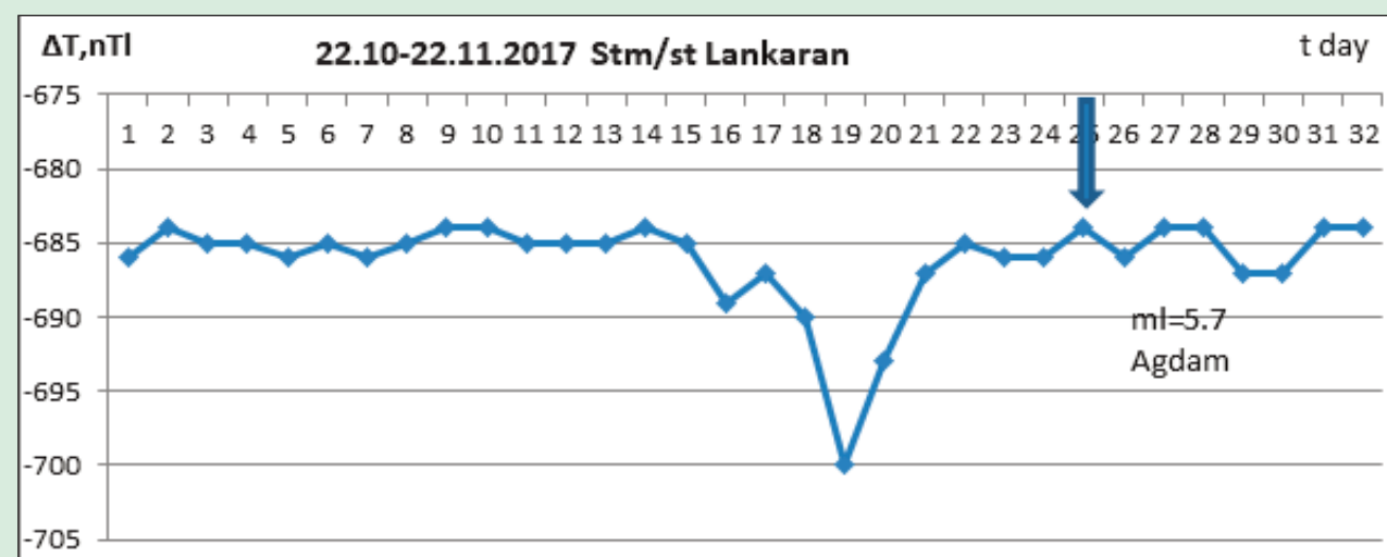
Şəkil 2. Ağdam ( m_l = 5.7 , 15.11.2017) zəlzələsi zamanı müşahidə olunan seysmomaqnit effekt
